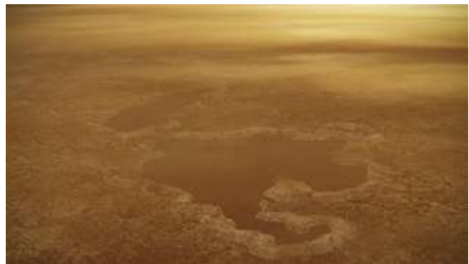
Methanseen auf der Oberfläche des Saturnmonds Titan
